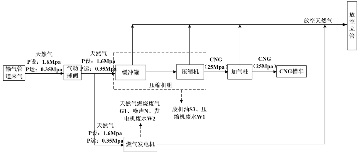
图 2.8-1 项目运营期生产工艺流程及产污环节图
