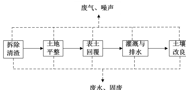
图 2.9-1 退役期拆除工程及土地复垦工艺流程图
